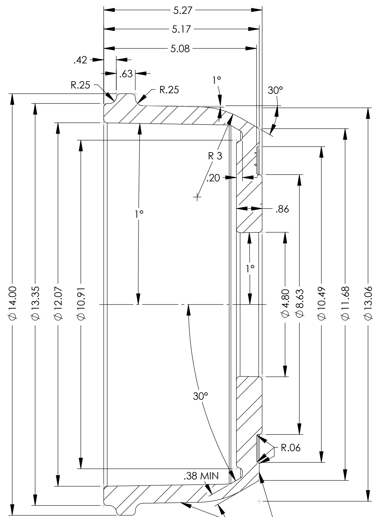
SECTION A-A SCALE 1 : 2
