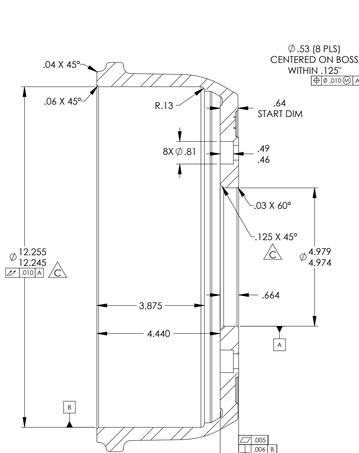
SECTION B-B SCALE 1 : 2
